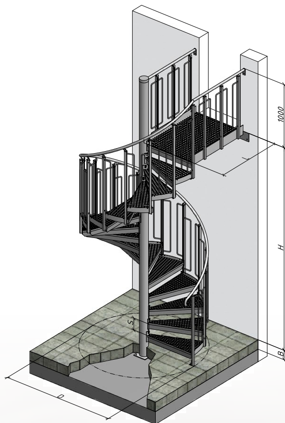
Stufe mit Gitterrost Maschenweite 30/10 mm rutschhemmend
