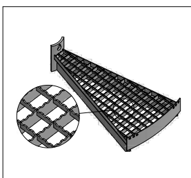
Stufe mit Gitterrost Maschenweite 30/30 mm rutschhemmend
