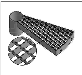
Stufe mit Gitterrost Maschenweite 30/30 mm
